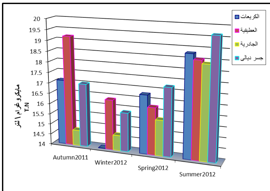
الشكل (١٨) التغيرات الفصلية لقيم النتروجين الكلي في مواقع الدراسة .
