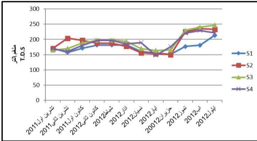
ملحق (١٢) المتغيرات الشهرية للمواد الذائبة الكلية
