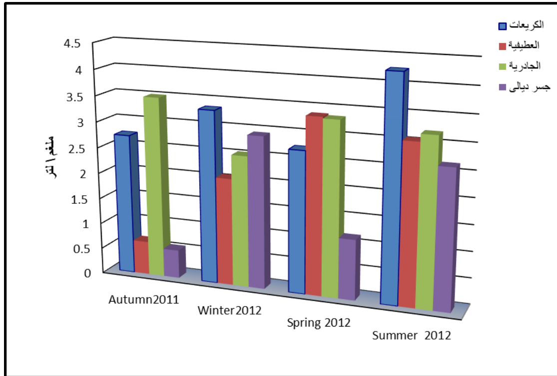
الشكل (١٦) التغيرات الفصلية لقيم المتطلب الحيوي للاوكسجين في مواقع الدراسة.
