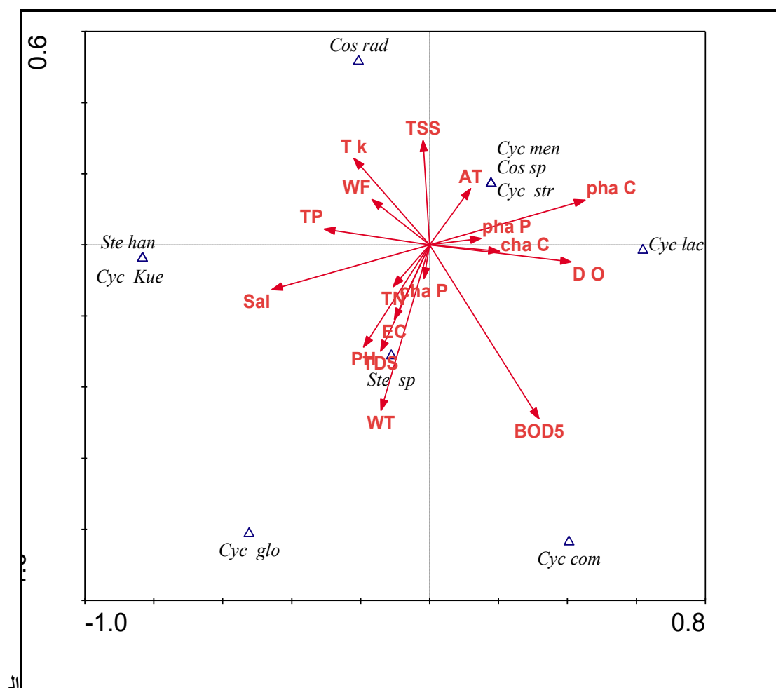
شكل (٣٧) يوضح علاقة العوامل البيئية مع الطحالب العسوية(المركزية) المشخصة على نبات الشمبلان
