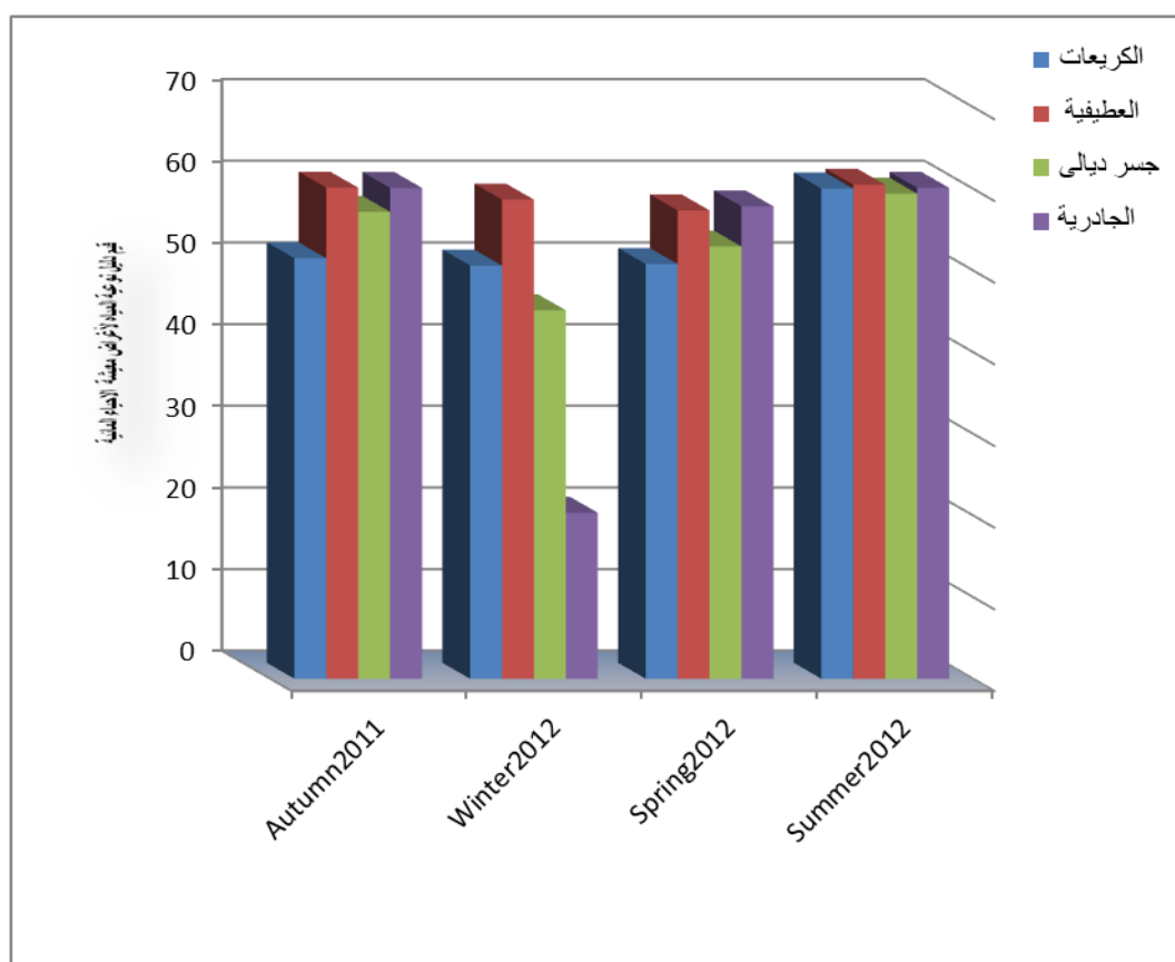
شكل (٤٣) قيم دليل نوعية المياه لأغراض معيشة الأحياء المائية في محطات الدراسة أثناء فصول ٢٠١١ - ٢٠١٢ .
